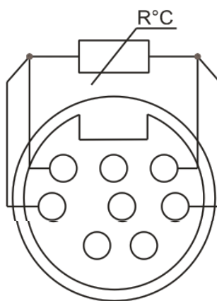
Рисунок 7.2 Входной преобразователь – термопреобразователь сопротивления
